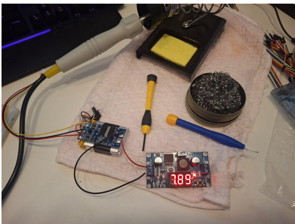
Figura 2 - Buck Converter mostrando a tensão da bateria, Input.
