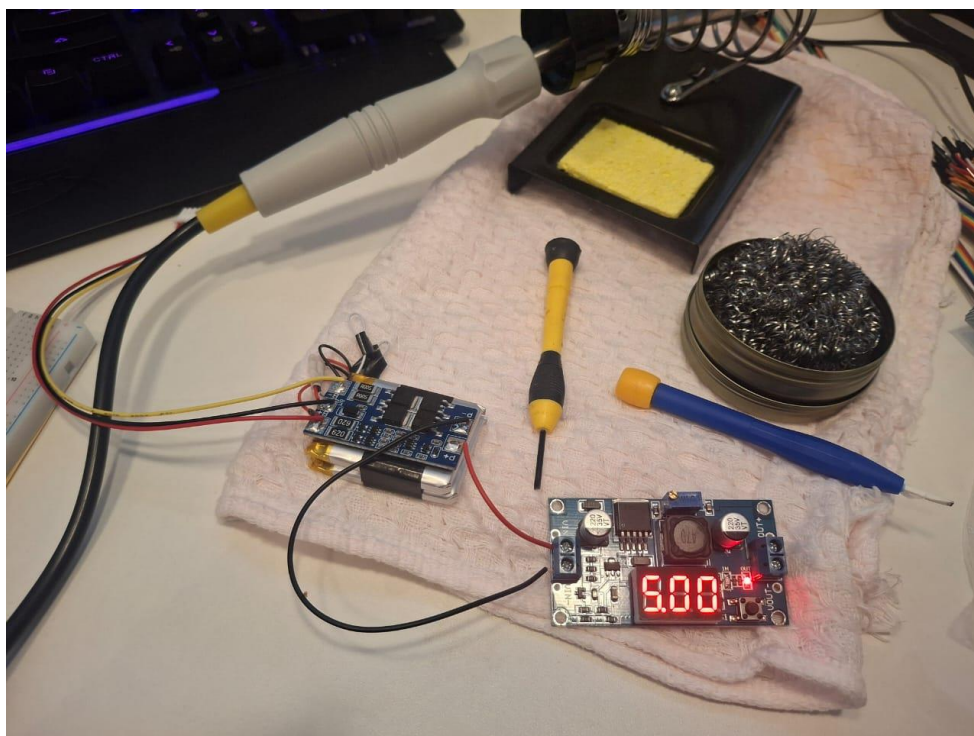
Figura 1 - Buck Converter mostrando a tensão que vai para a ESP, Output.
